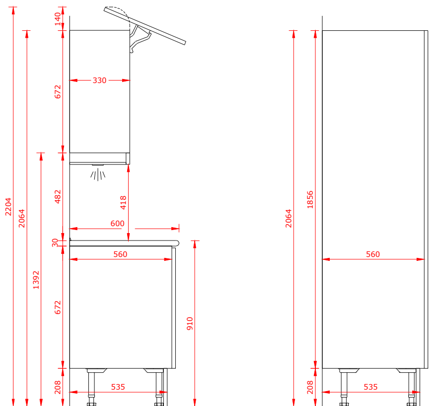
Målskitse Maßzeichnung Dimensional drawing
